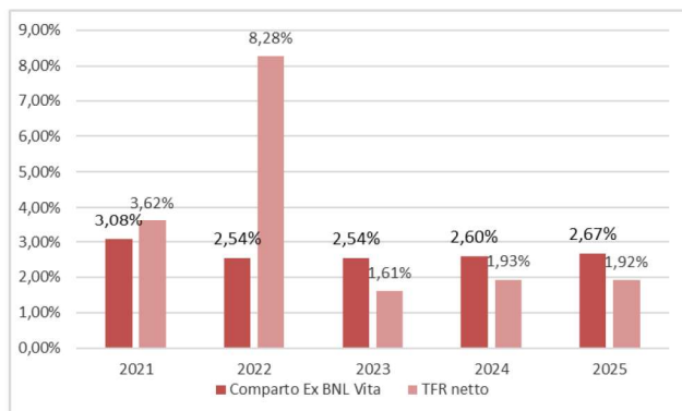
Tav. 5. Rendimento medio annuo composto
