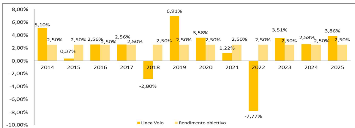
Tav. 5. Rendimento medio annuo composto **
